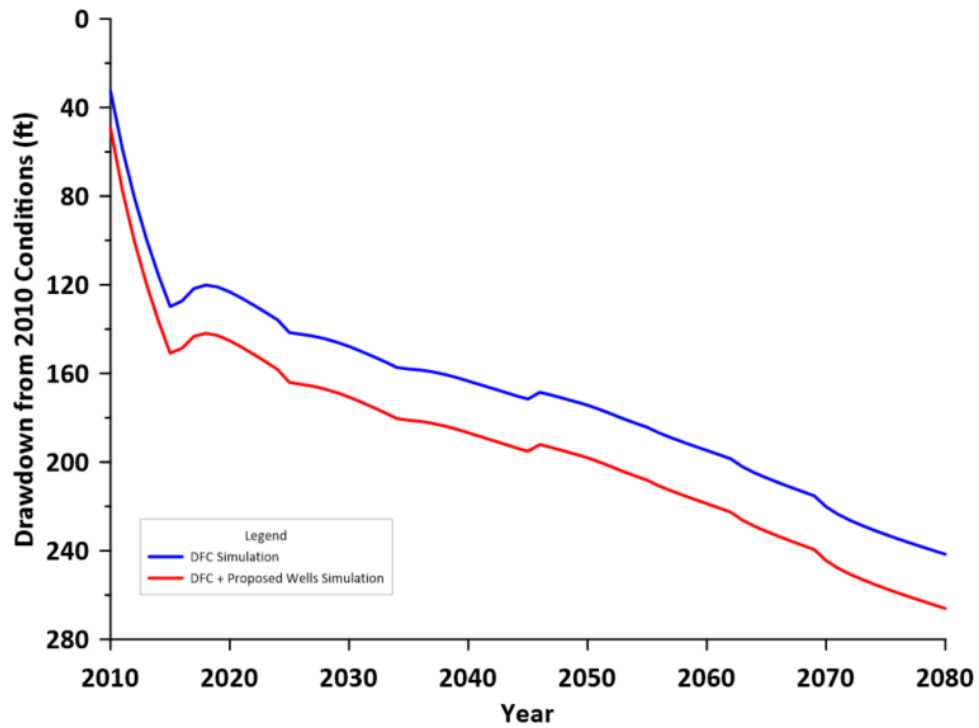
HAGM Drawdown (Jasper) Layer 1, Row 33, Column 95 (BWLL-4025)
